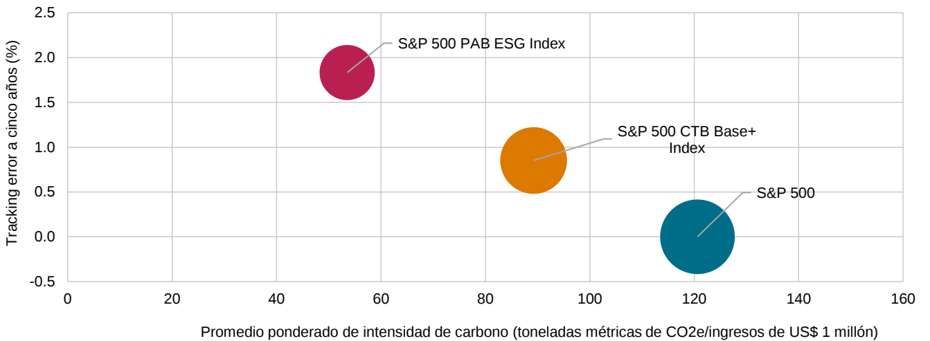
Figura 6: promedio ponderado de intensidad de carbono versus tracking error a cinco años
