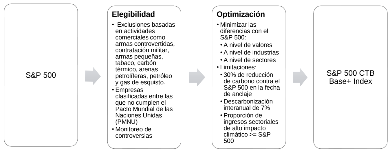
Figura 2: metodología del índice 2
