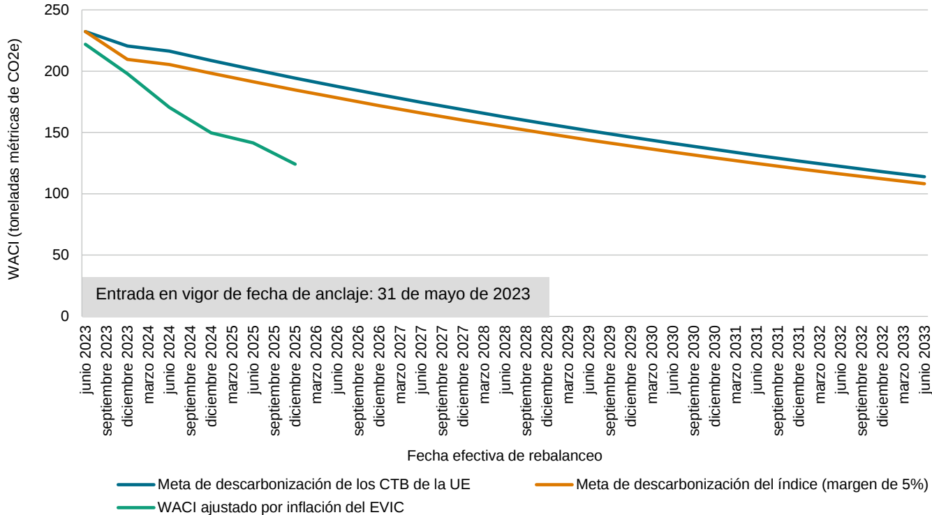
Figura 3: objetivo de descarbonización del S&P 500 CTB Base+ Index
