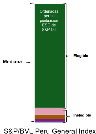
Figura 1: construcción del índice
